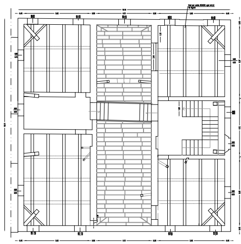
PIANTA PRIMO SOTTOTETTO
