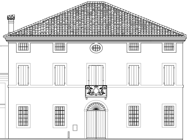
PROSPETTO FRONTALE
