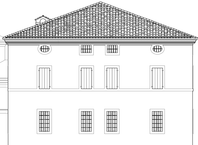
PROSPETTO LATERALE VERSO IL CONFINE
